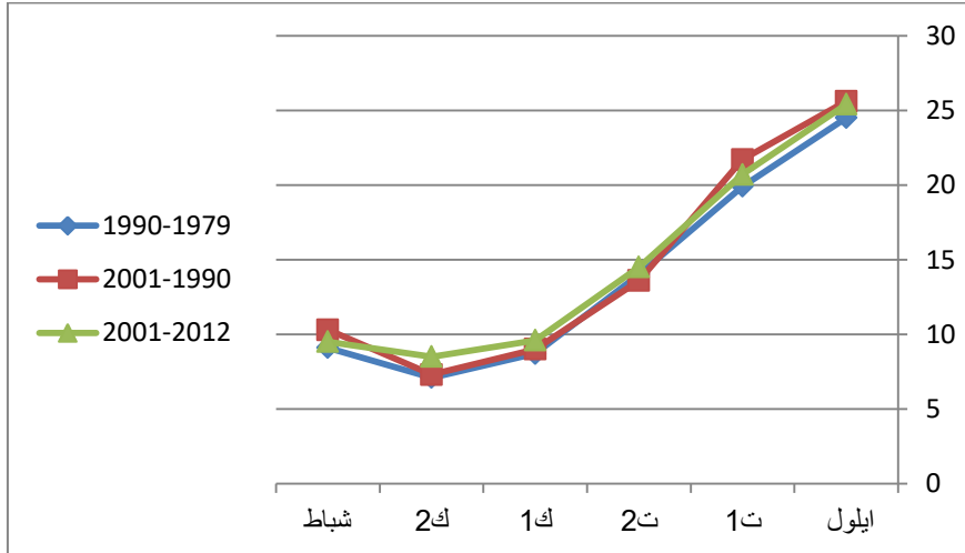
شكل (٥) اتجاه تغير معدلات درجات الحرارة الصغرى (م) للموسم الزراعي الشتوي للمدة (١٩٩٠-٢٠٢٢)
